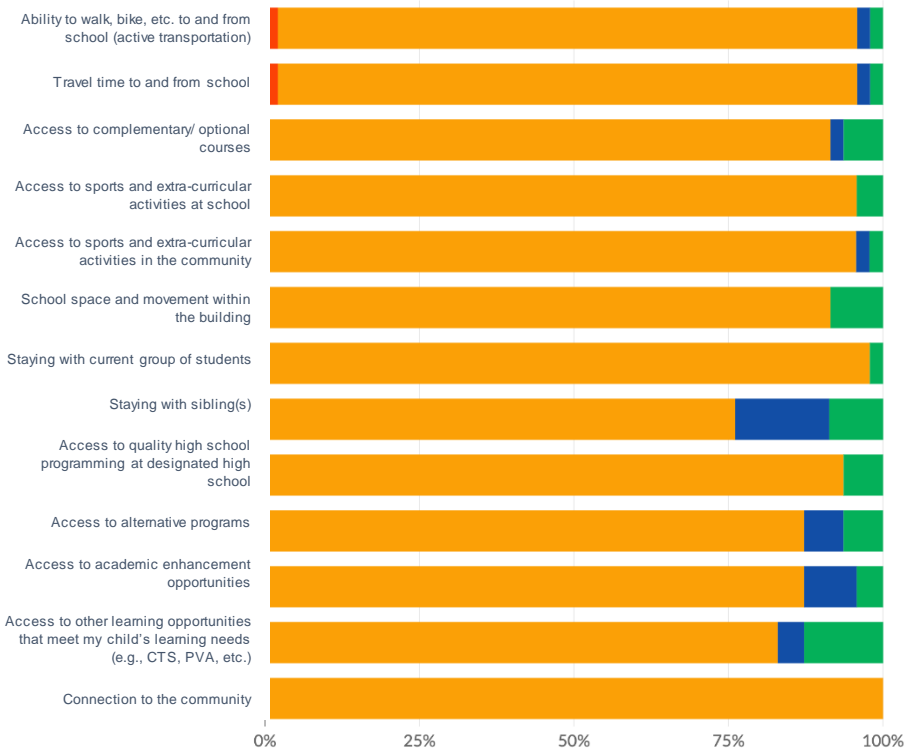
Scenario A
