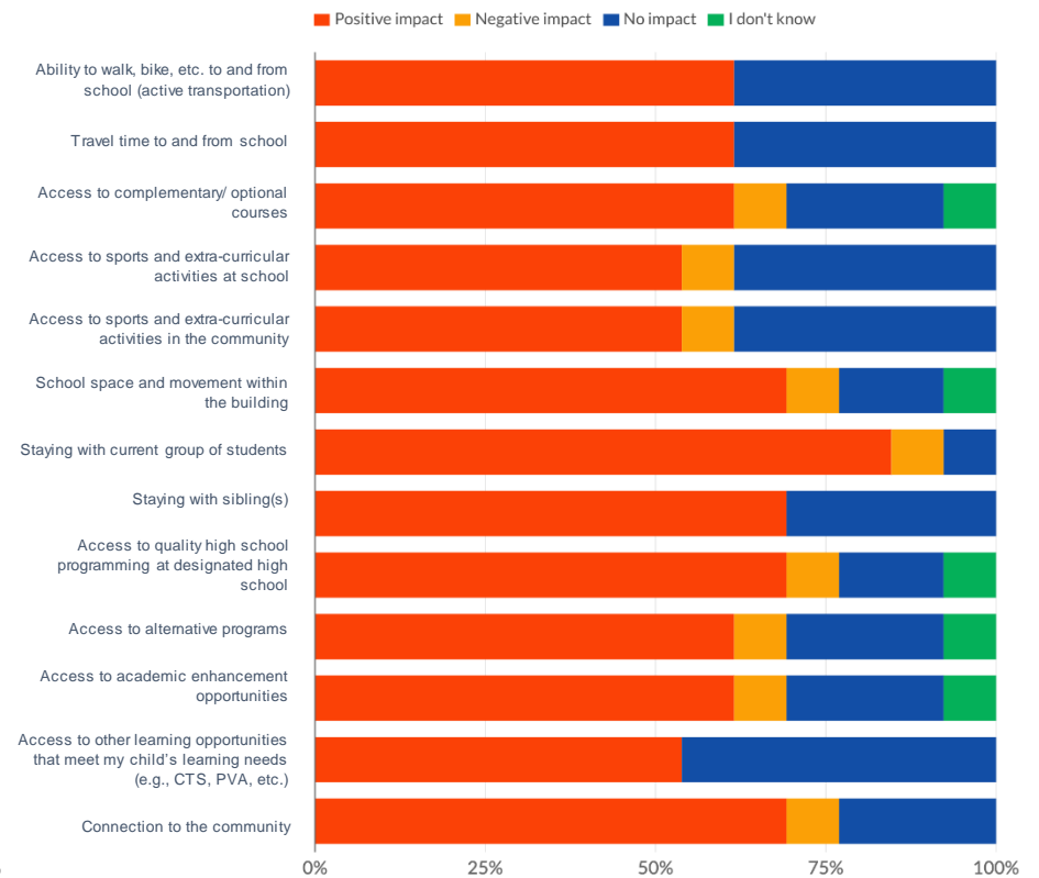
Scenario B
