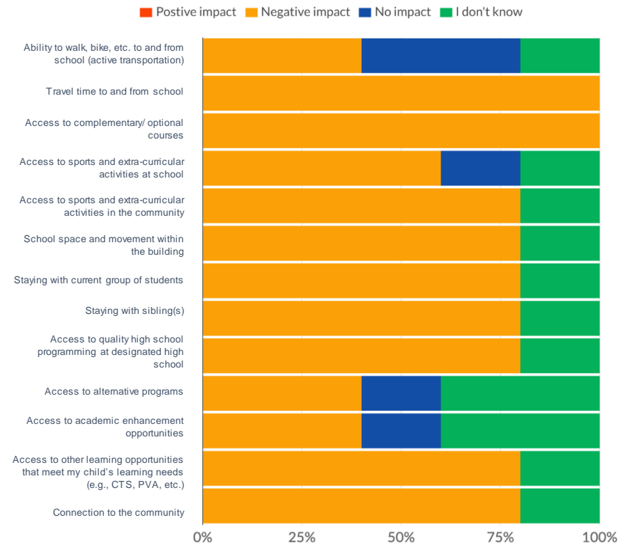
Scenario B
