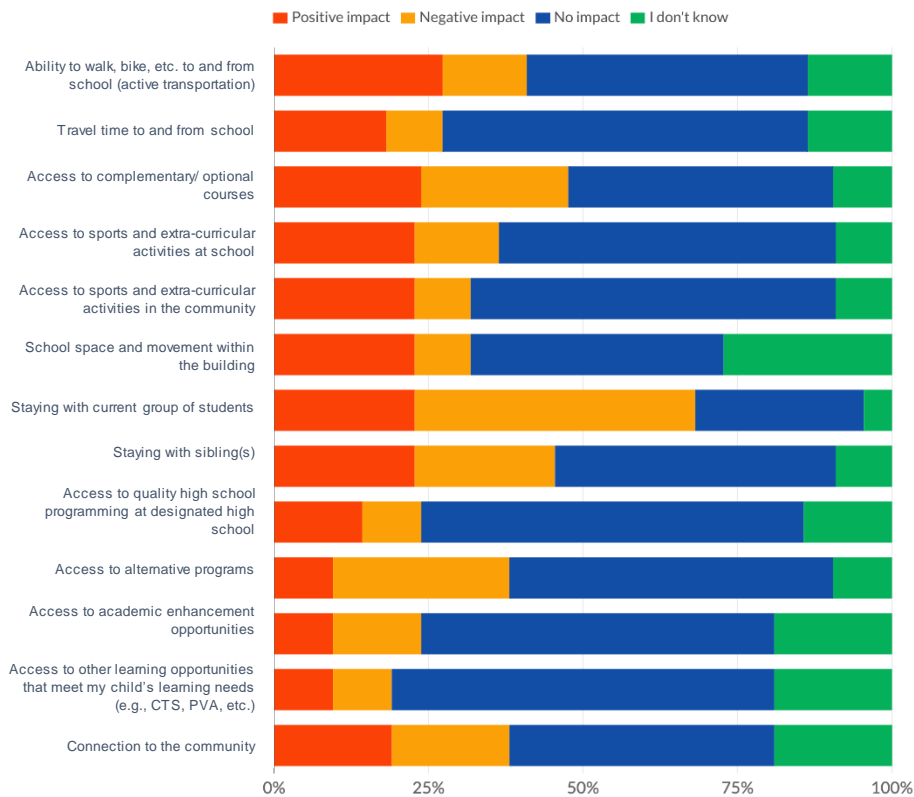
Scenario A
