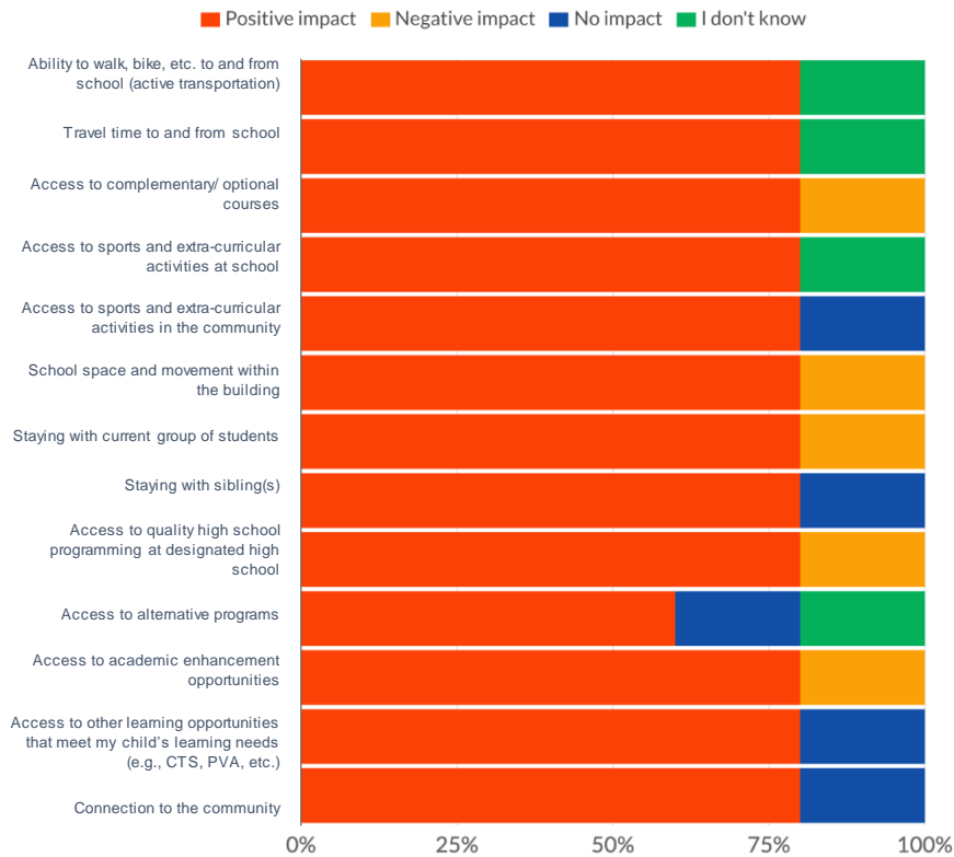
Scenario A
