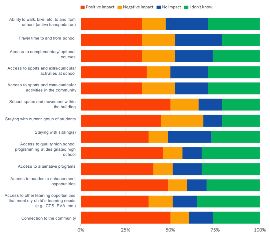
Scenario B
