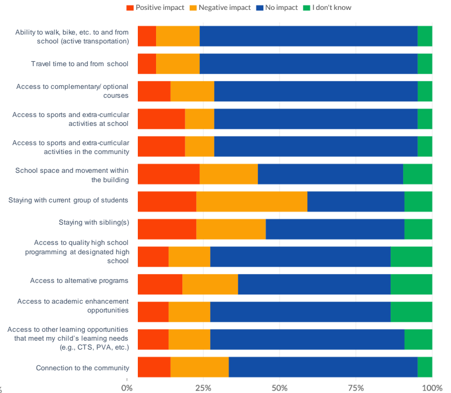
Scenario B
