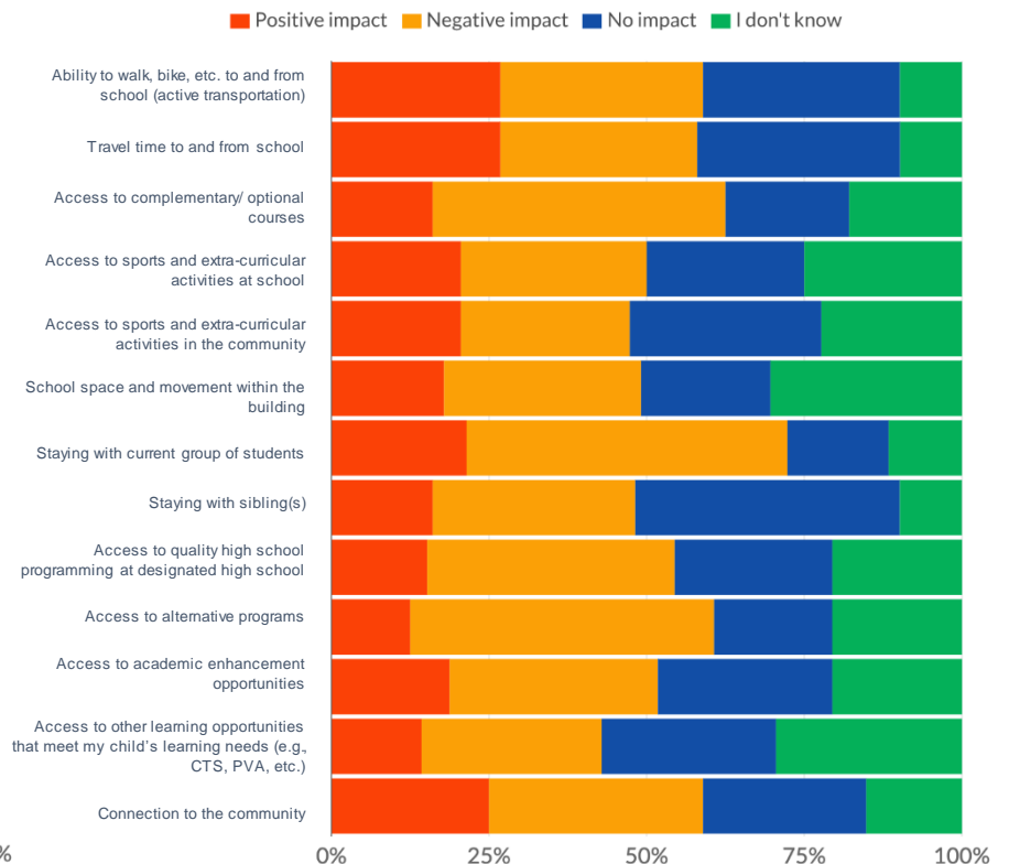
Scenario B
