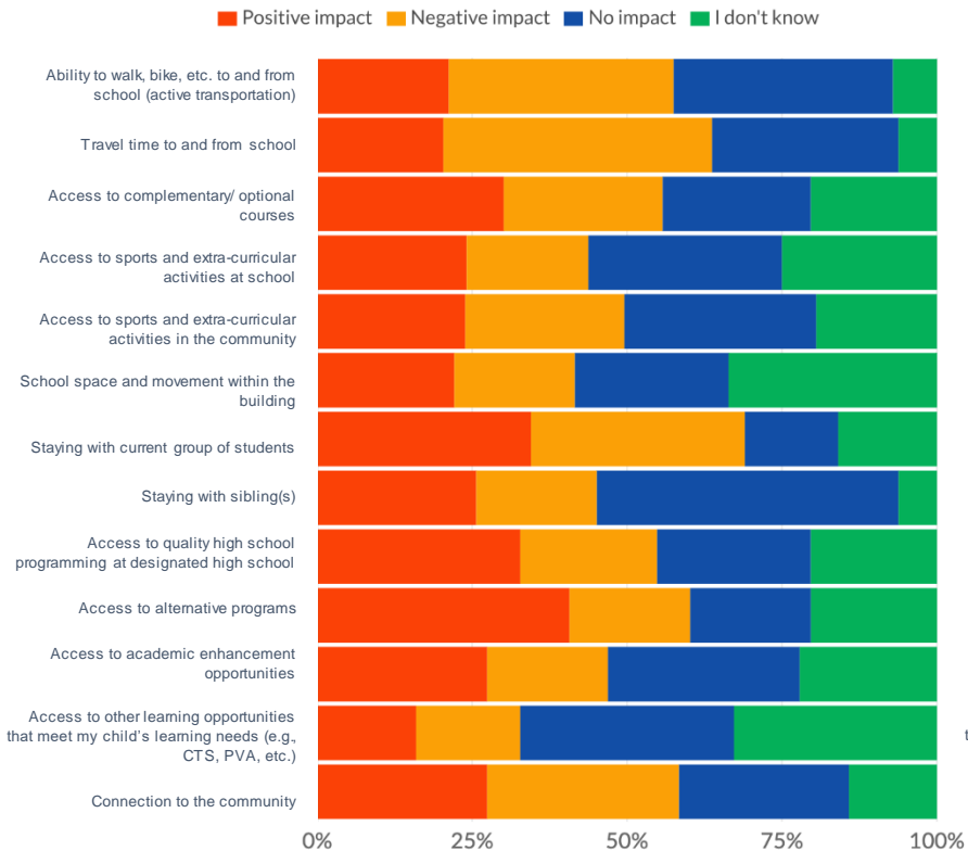
Scenario A
