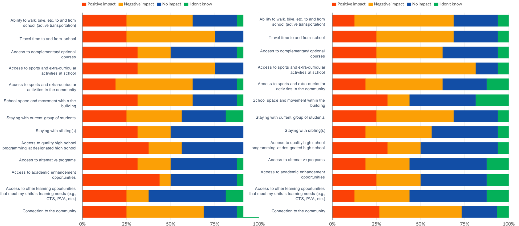
Scenario A
