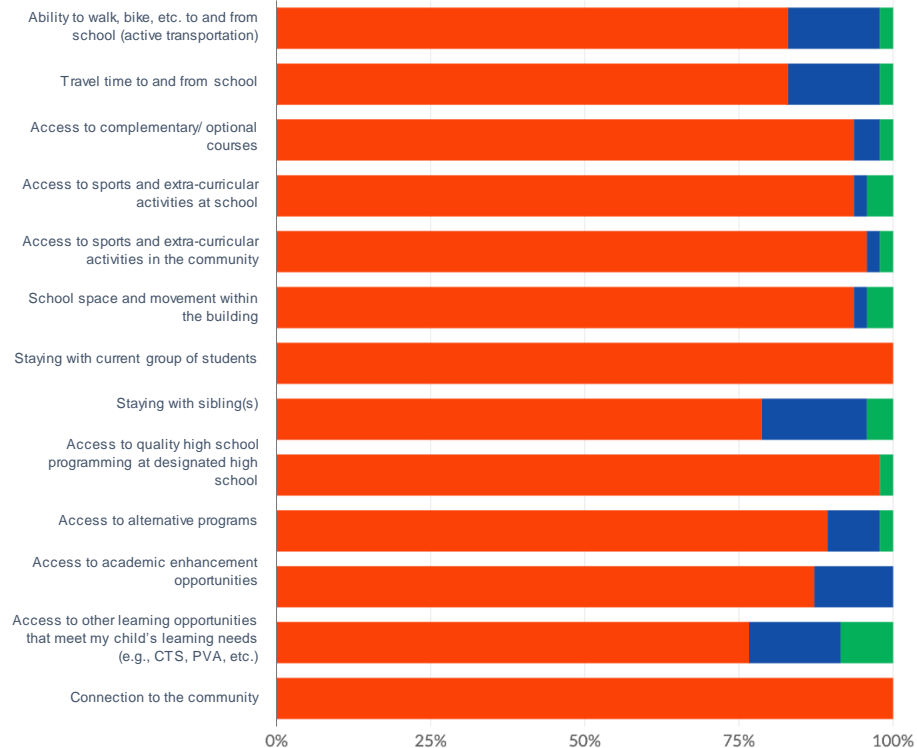
Scenario B
