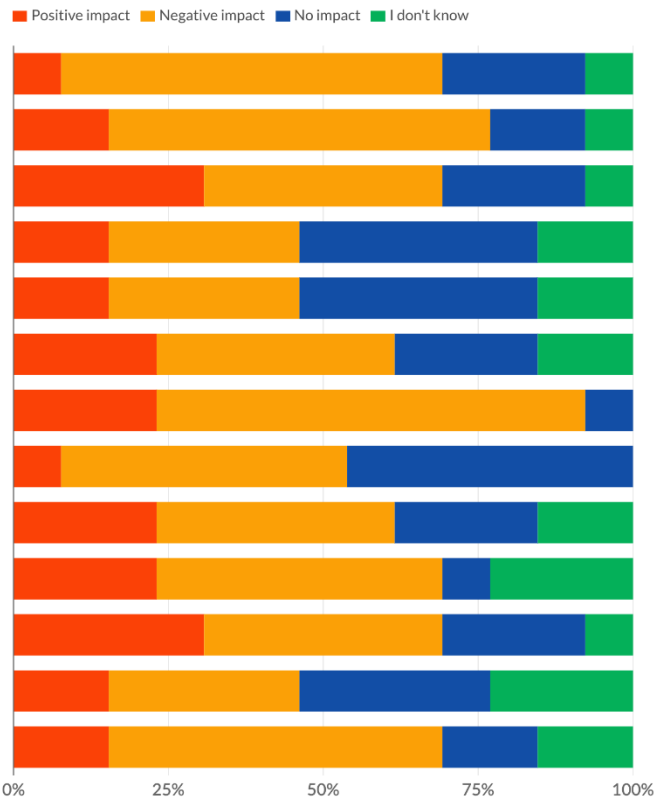
Scenario A
